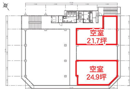
5階平面図
