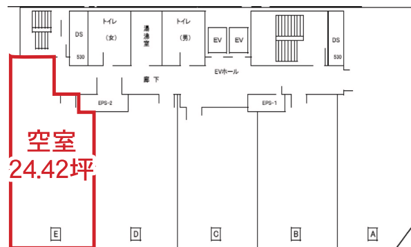
3 階平面図
