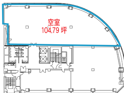
6階平面図
